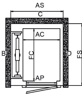
Acceso Simple Lateral
