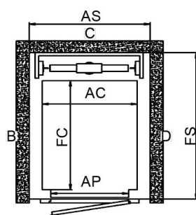
Acceso Simple Posterior
