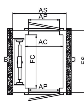
Acceso Doble 2 x 180°
