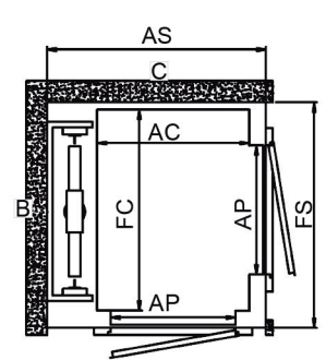
Acceso Doble 2 x 90°
